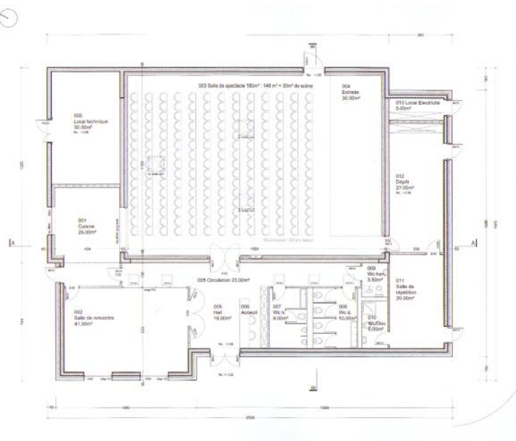
Plan de la nouvelle salle polyvalente à la Villa Tacchini
